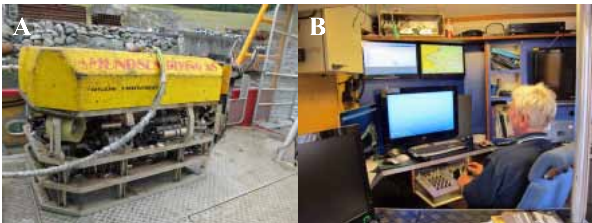
Figur 13 A. ROV, type Argus Mariner 1. B. Mannskap fra Amundsen Diving AS styrer ROV'en i kontrollrom på båten MS Scuba.
